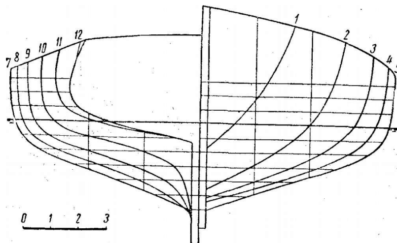
Теоретические шпангоуты «Спрея».
