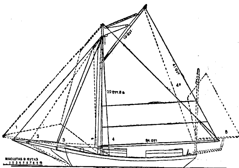
Парусное вооружение «Спрея»:
