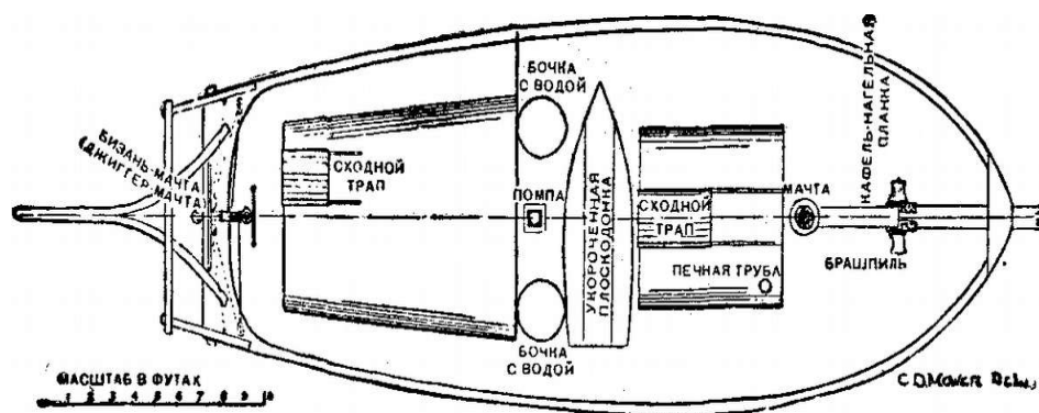
План палубы „Спрея“
