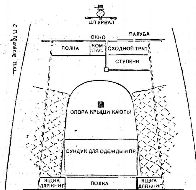
План каюты на „Спрее“
